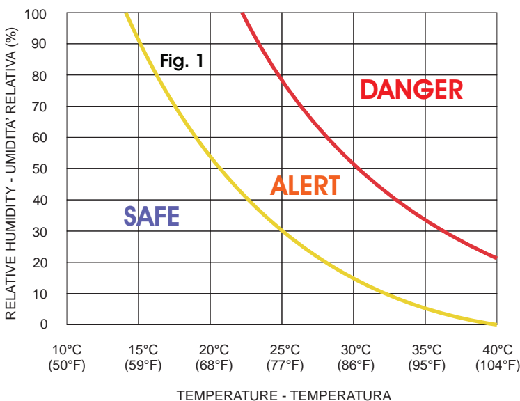
Fig 1. Thermal comfort zones.
